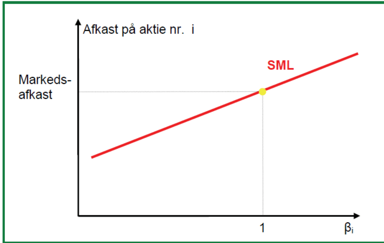
Figur 6.15 Aktiemarkedslinje
