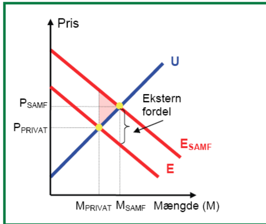
Figur 6.3 Eksterne fordele
